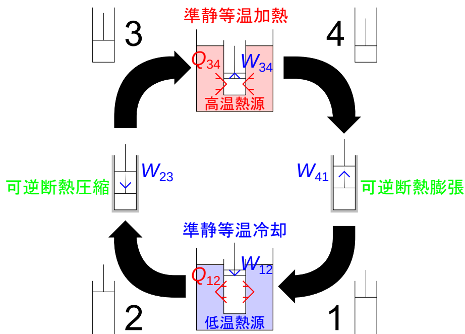
図 C.1 可逆サイクル (カルノーサイクル)
