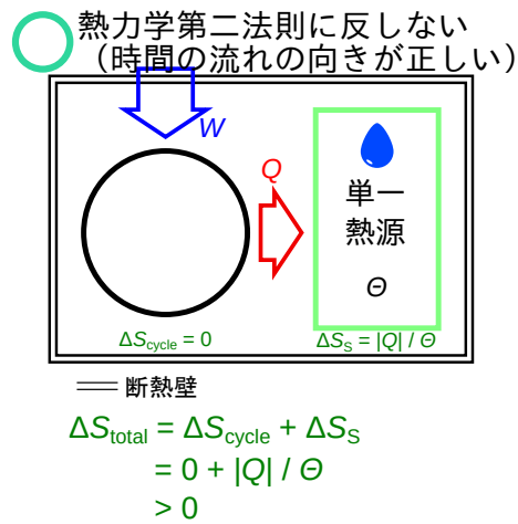
図 2.10 熱源とトムソンの表現
