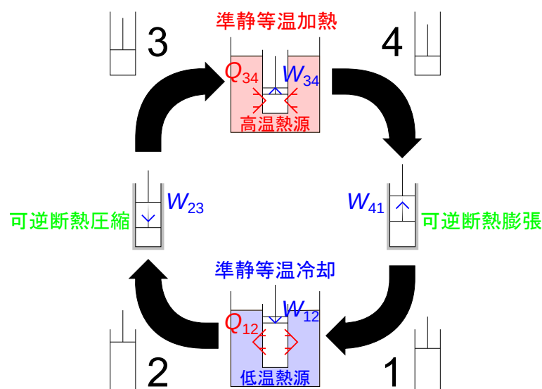
図 5.18 カルノーサイクル
