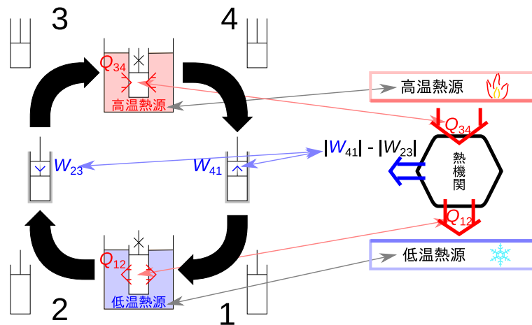
図 5.9 熱機関の表示
