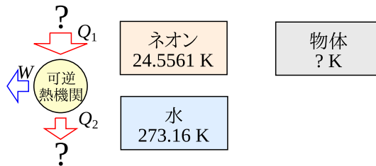
図 3.5 温度の測定
