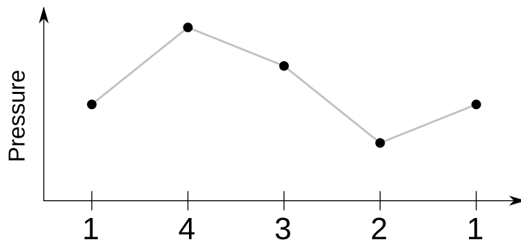
図 5.12 ピストンでのヒートポンプとして動作するサイクルの圧力変化
