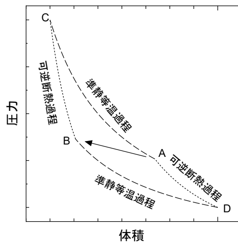
図 B.11 可逆過程による経路の PV 線図
