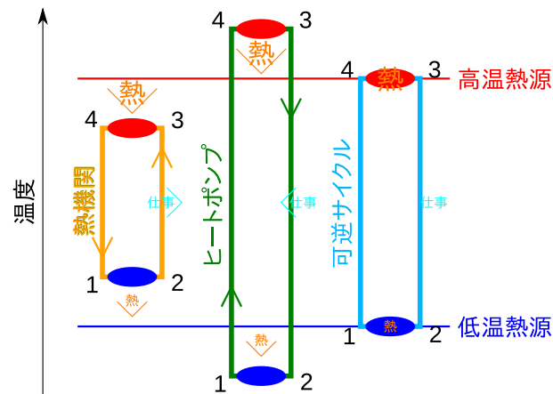
図 5.16 熱機関とヒートポンプにおける熱源との温度の関係
