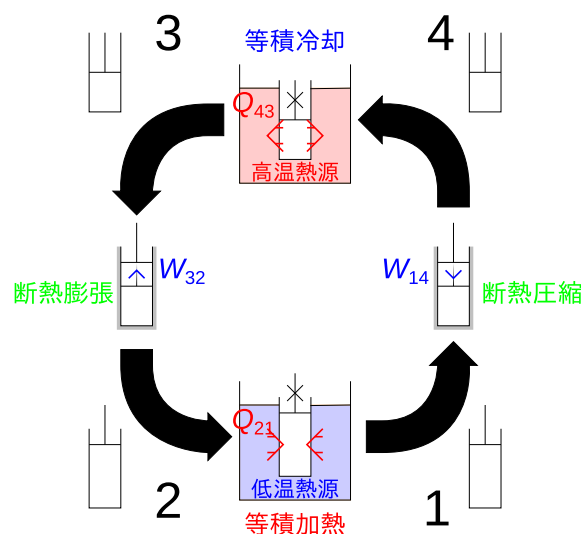
図 5.11 ピストンでのヒートポンプとして動作するサイクル
