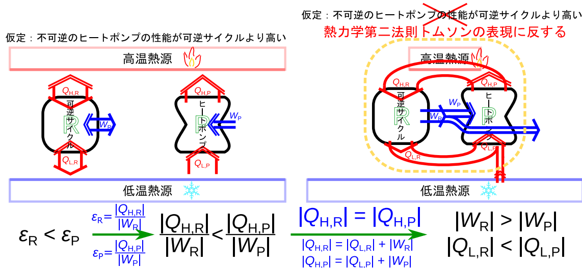
図 B.9 可逆サイクルと不可逆ヒートポンプの比較 (トムソンの表現)
