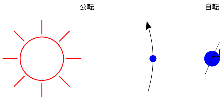
図 1.8 回転による運動エネルギー
