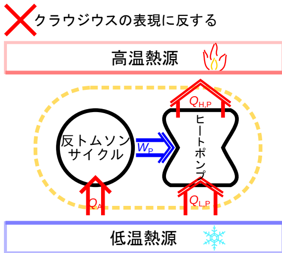
図 B.3 反トムソンの表現から反クラウジウスの表現
