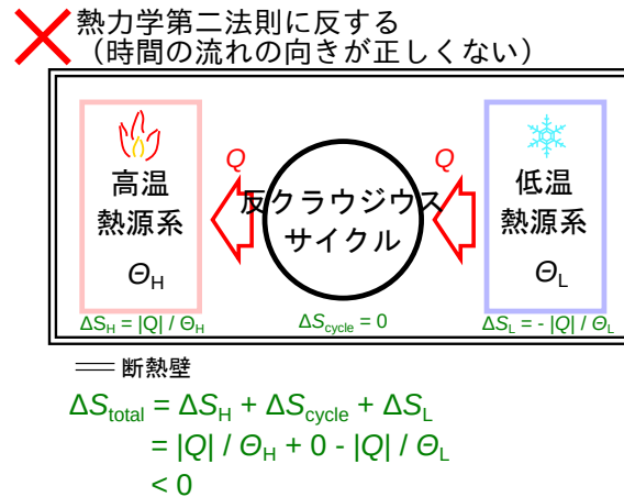
図 2.14 エントロピーと反クラウジウスサイクル
