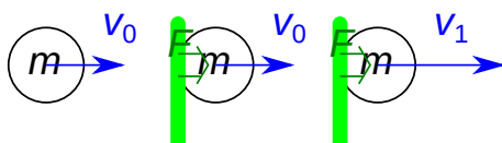
図 1.7 運動エネルギー
