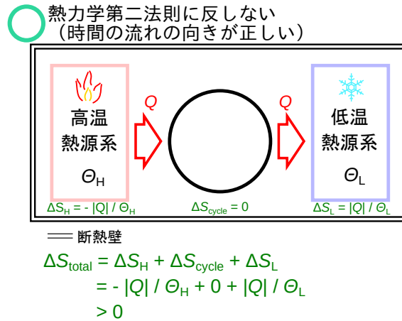
図 2.13 エントロピーとクラウジウスの表現
