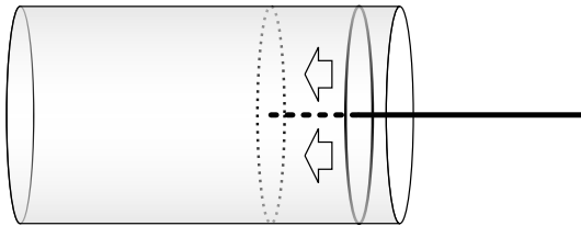
図 1.5 並進運動による仕事
