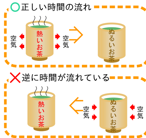
図 2.2 熱の伝わり
