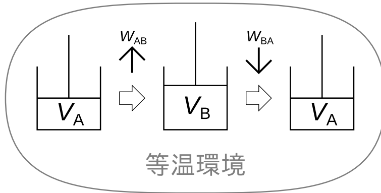
図 5.19 等温過程
