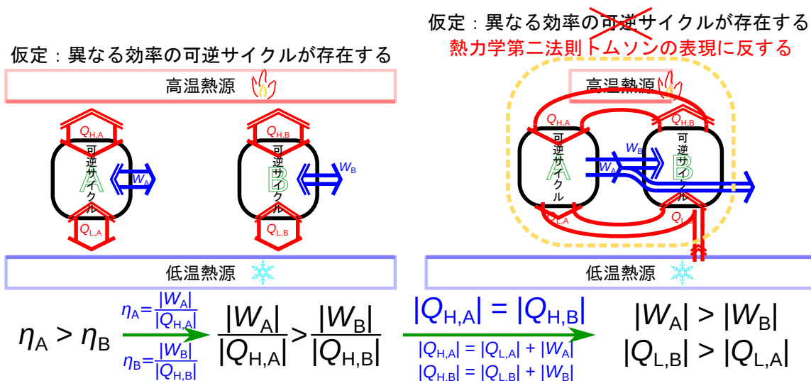
図 2.6 可逆サイクルの比較
