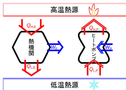
図 1.15 熱機関とヒートポンプ
