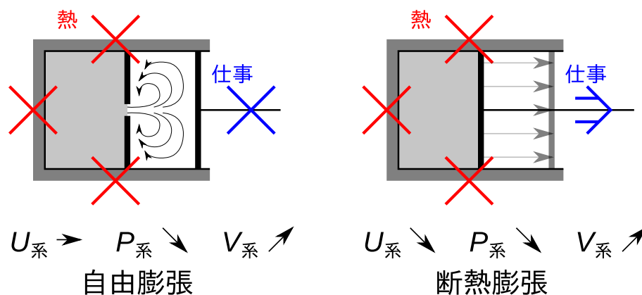
図 D.5 自由膨張過程
