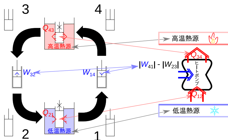
図 5.14 ヒートポンプの表示
