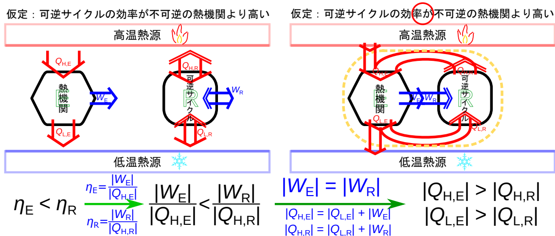
図 B.8 可逆サイクルと不可逆サイクルの比較
