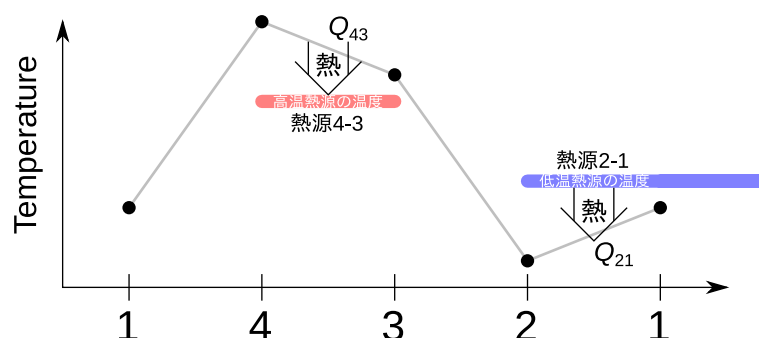
図 5.13 ピストンでのヒートポンプとして動作するサイクルの温度変化
