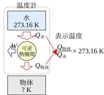
図 3.6 温度の測定方法
