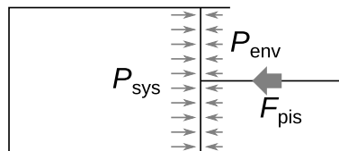
図 D.3 力の釣り合い（系の圧力が高い場合）
