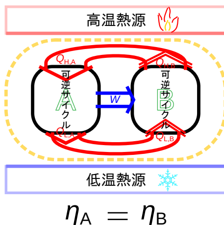
図 2.7 効率の等しい可逆熱機関（可逆ヒートポンプ）
