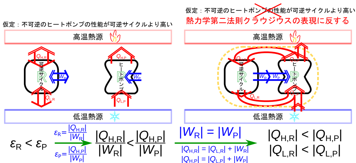
図 B.10 可逆サイクルと不可逆ヒートポンプの比較 (クラウジウスの表現)
