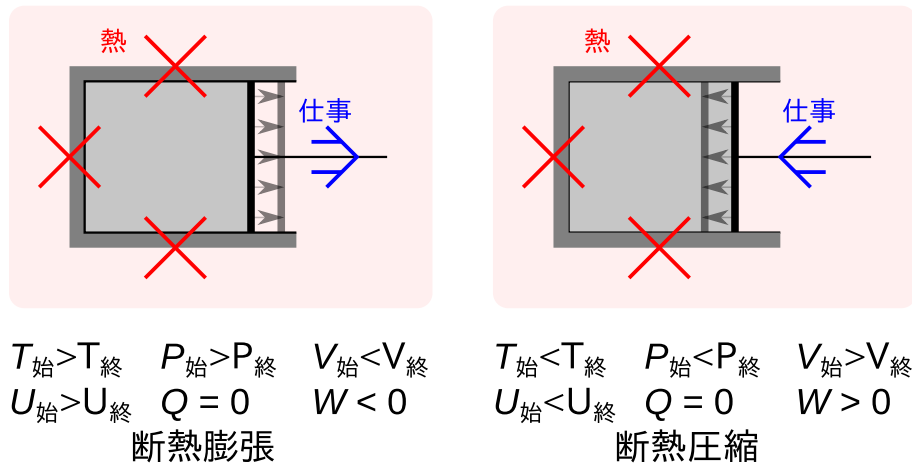
図 5.2 断熱過程
