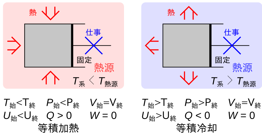
図 5.3 等積過程
