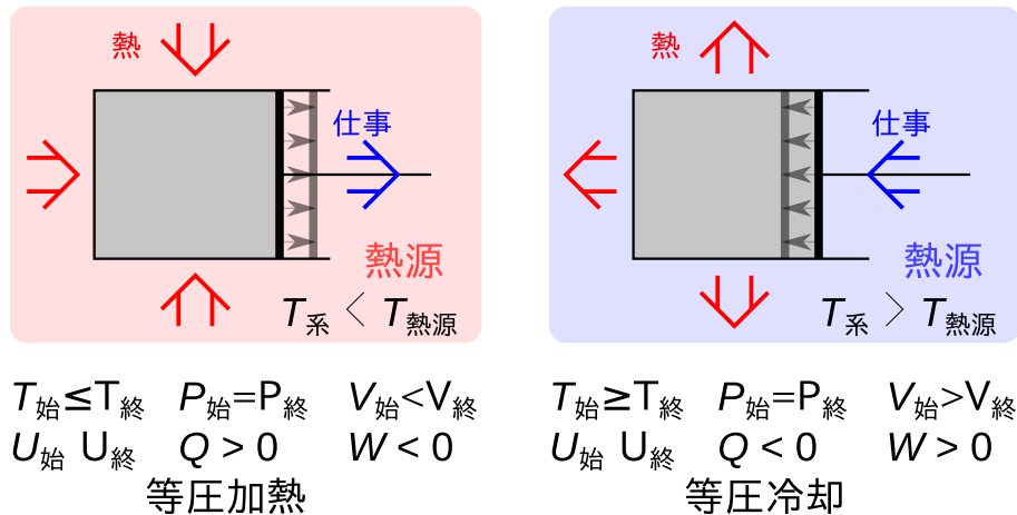
図 5.5 等圧過程
