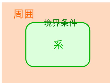
図 1.1 系と周囲
