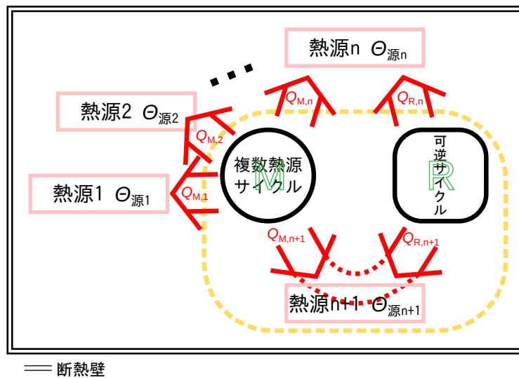
図 2.15 複数熱源
