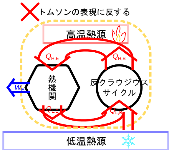
図 B.4 反クラウジウスの表現から反トムソンの表現
