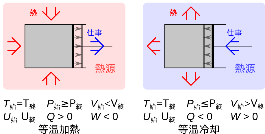
図 5.4 等温過程
