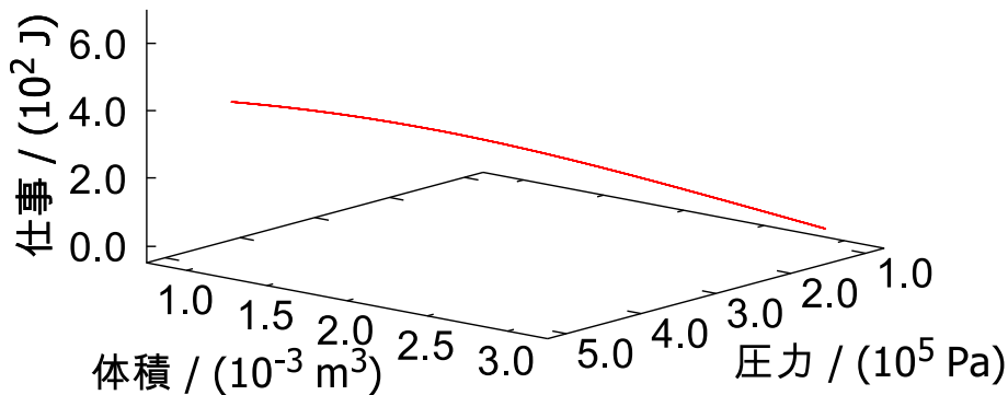
図 D.2 媒介変数表示による仕事
