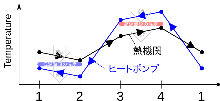
図 5.15 熱機関とヒートポンプにおける温度変化
