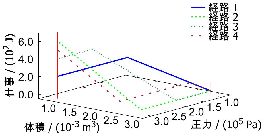
図 D.1 経路による仕事の変化
