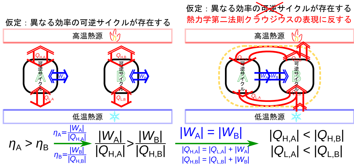
図 B.5 可逆サイクルの比較
