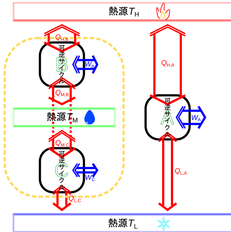
図 2.9 可逆熱機関の効率
