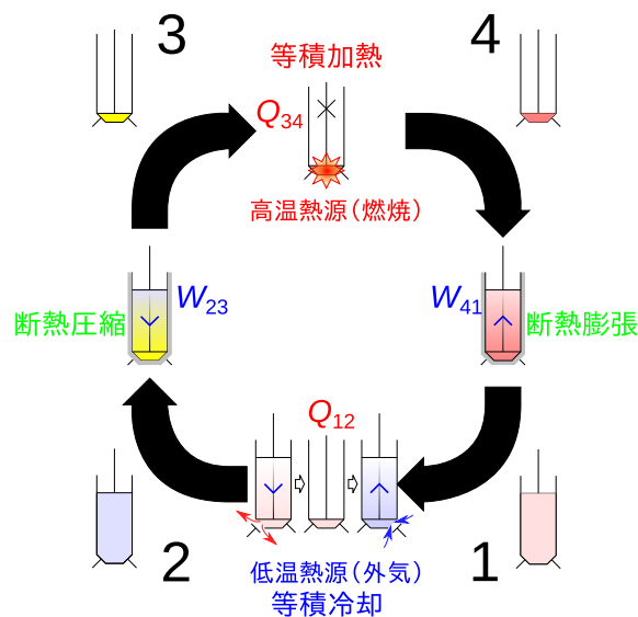
図 5.10 オットーサイクル
