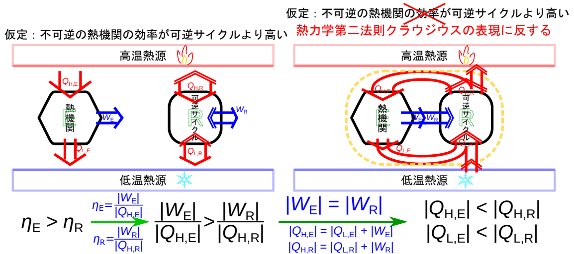
図 B.7 可逆熱機関と不可逆熱機関の比較
