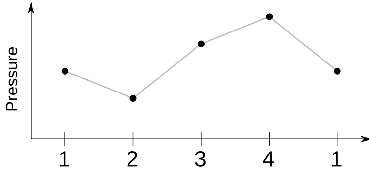
図 5.7 ピストンでの熱機関として動作するサイクルの圧力変化
