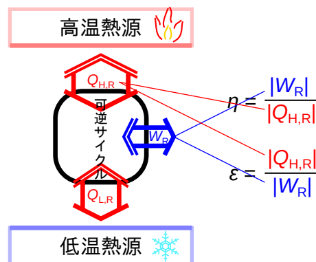
図 2.5 可逆サイクル
