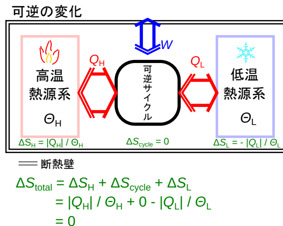
図 2.12 熱源と可逆サイクル
