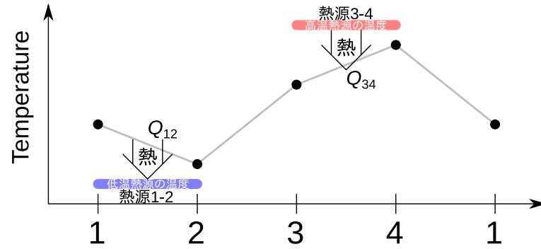
図 5.8 ピストンでの熱機関として動作するサイクルの温度変化
