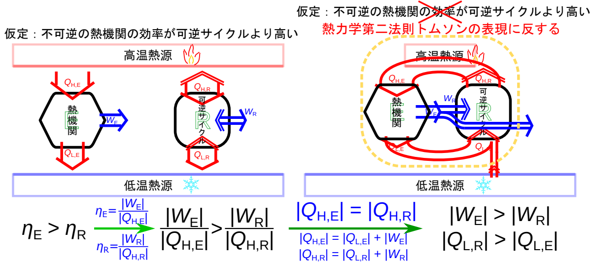
図 B.6 可逆サイクルと不可逆熱機関の比較
