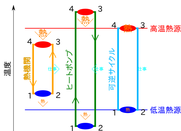
図 3.16 熱機関とヒートポンプにおける熱源との温度の関係
