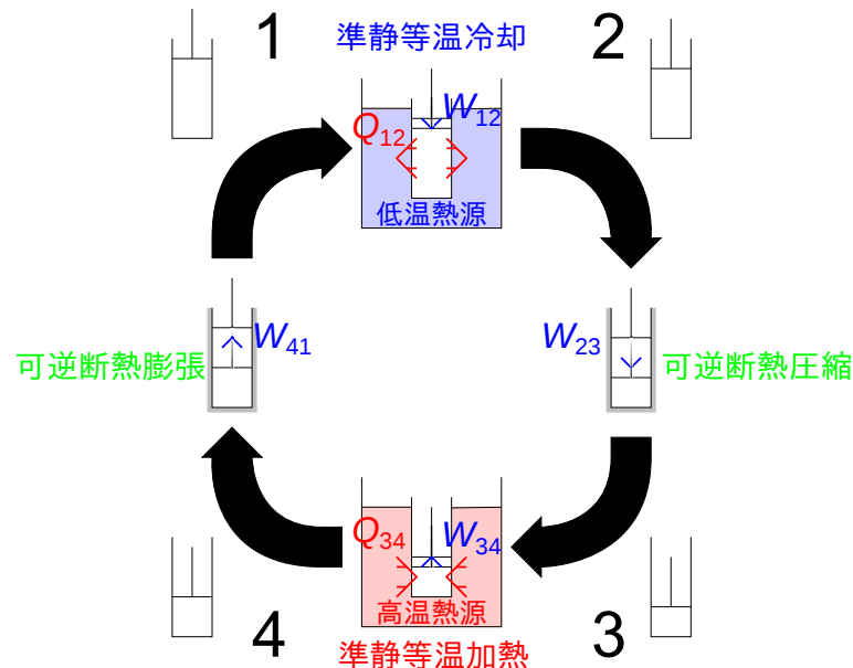
図 3.18 カルノーサイクル
