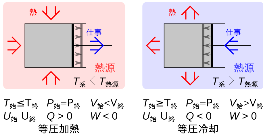
図 3.5 等圧過程
