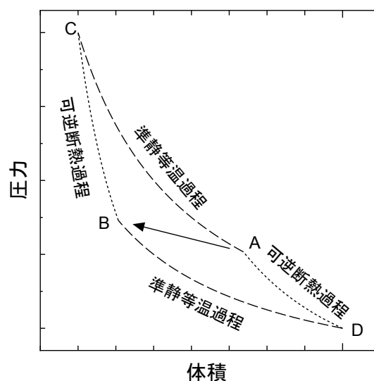
図 A.6 可逆過程による経路の PV 線図
