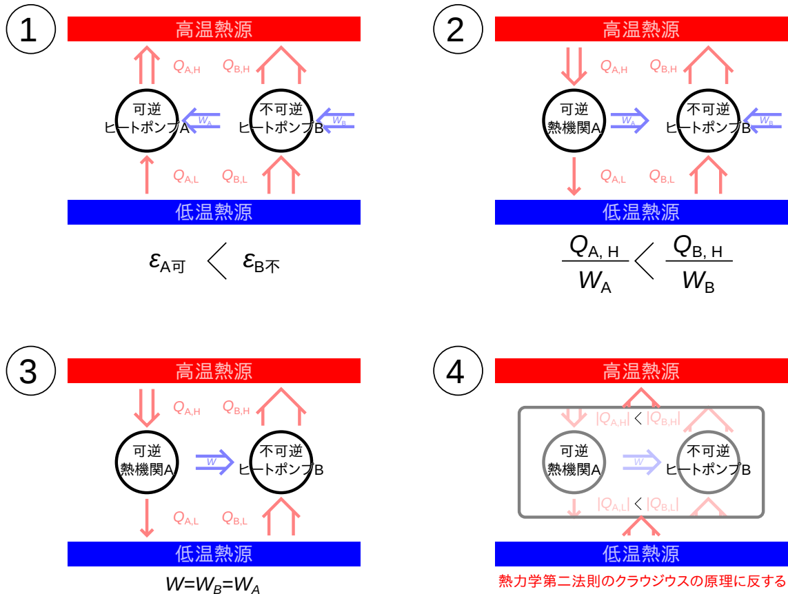
図 1.9 可逆ヒートポンプと不可逆ヒートポンプの比較
