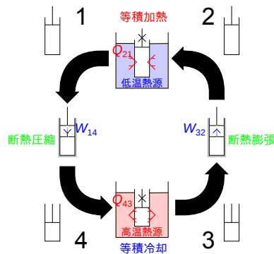
図 3.11 ピストンでのヒートポンプとして動作するサイクル
