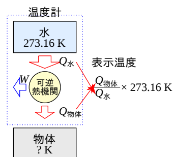
図 2.5 温度の測定方法
