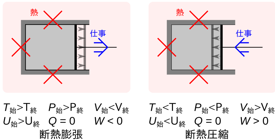
図 3.2 断熱過程
