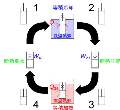
図 3.6 ピストンでの熱機関として動作するサイクル
