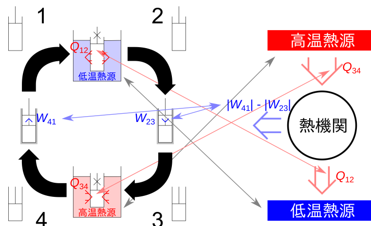
図 3.9 熱機関の表示
