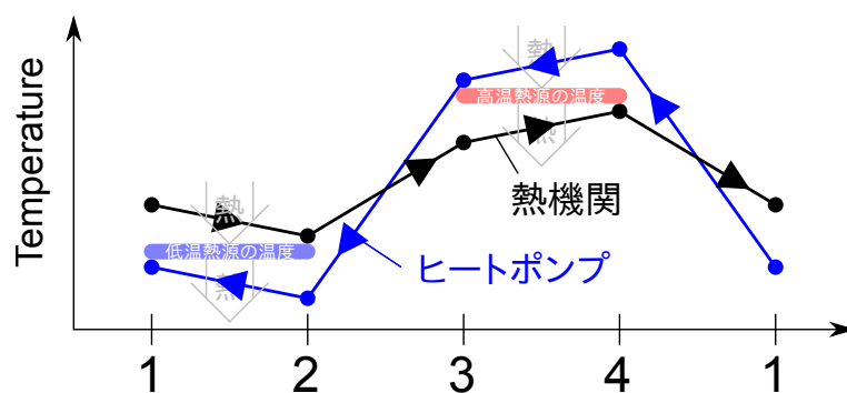
図 3.15 熱機関とヒートポンプにおける温度変化
