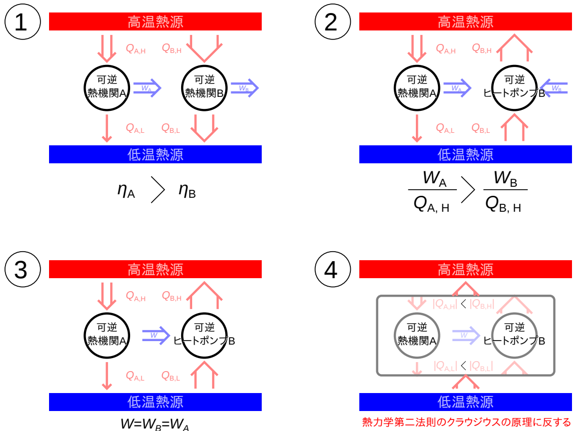
図 1.6 可逆熱機関（可逆ヒートポンプ）の比較
