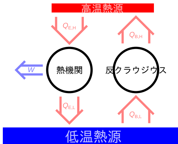
図 A.4 反クラウジウスの原理から反トムソンの原理
