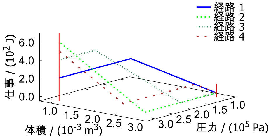
図 B.1 経路による仕事の変化
