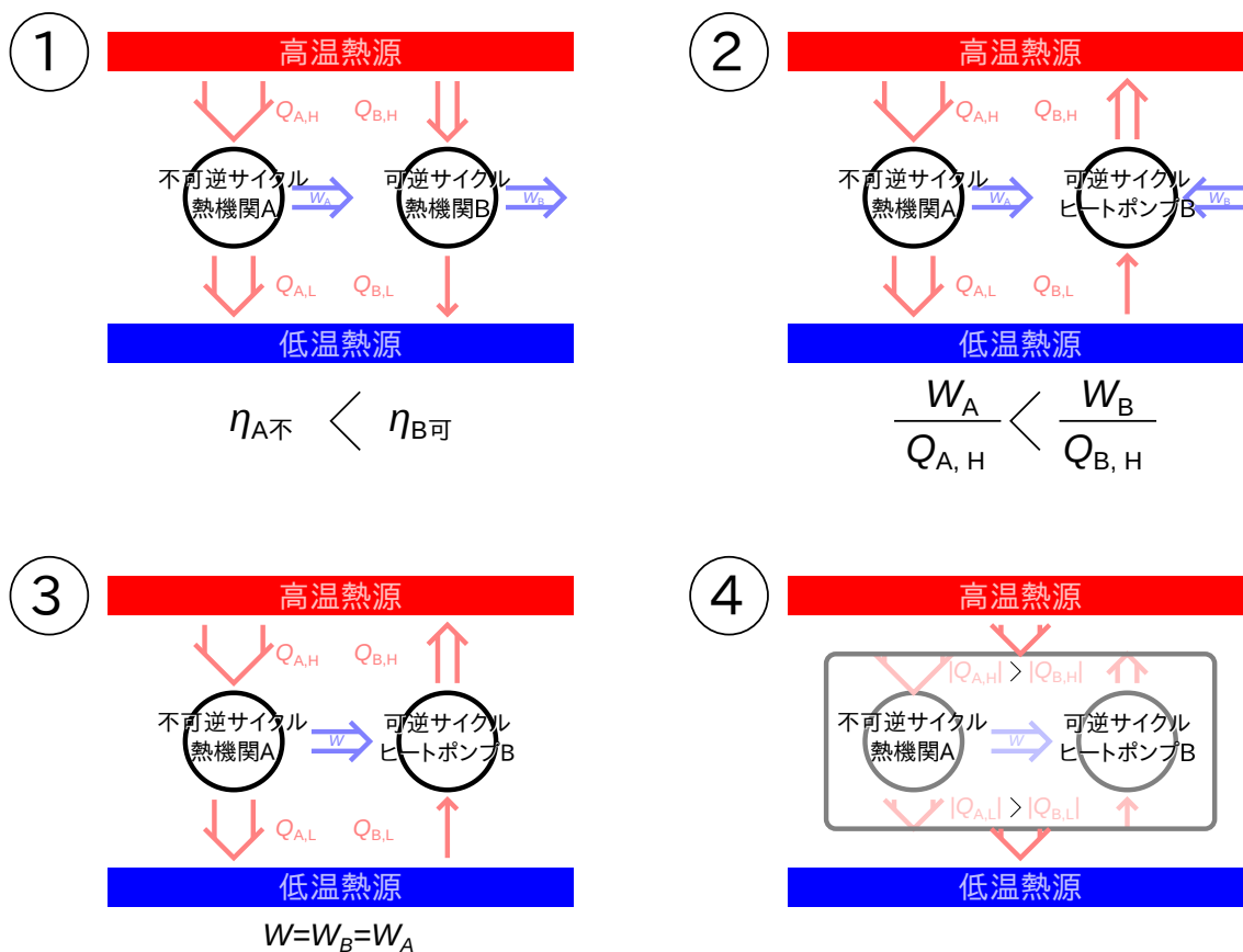
図 A.5 可逆サイクルと不可逆サイクルの比較
