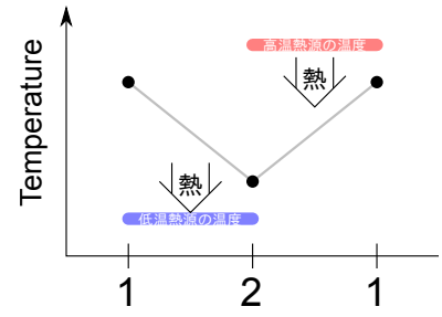
図 B.8 温度変化
