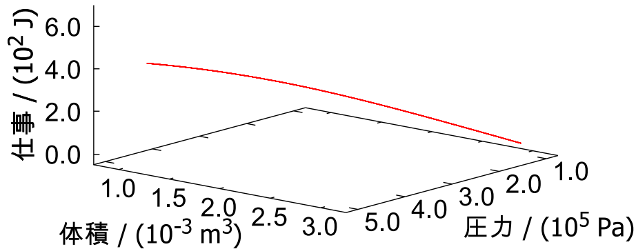
図 B.2 媒介変数表示による仕事
