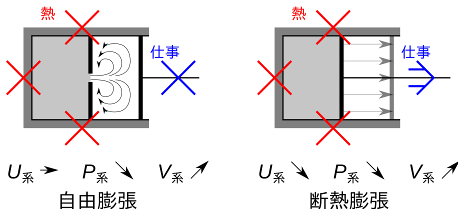
図 B.5 自由膨張過程
