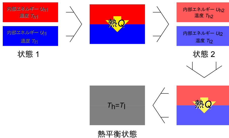
図 1.2 内部エネルギー・熱平衡
