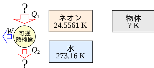
図 2.4 温度の測定
