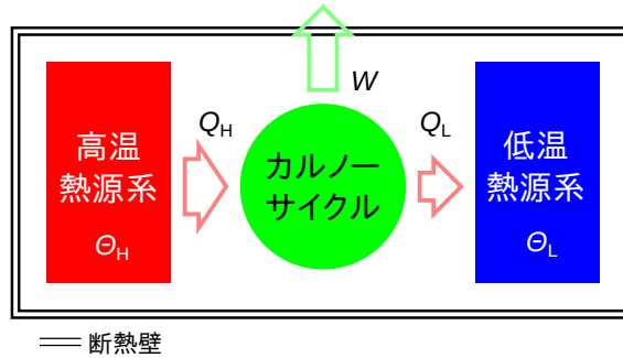
図 4.1 熱源とカルノーサイクル
