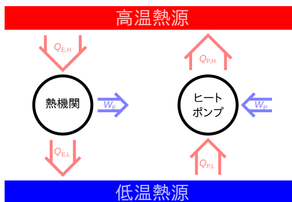
図 1.5 熱機関とヒートポンプ
