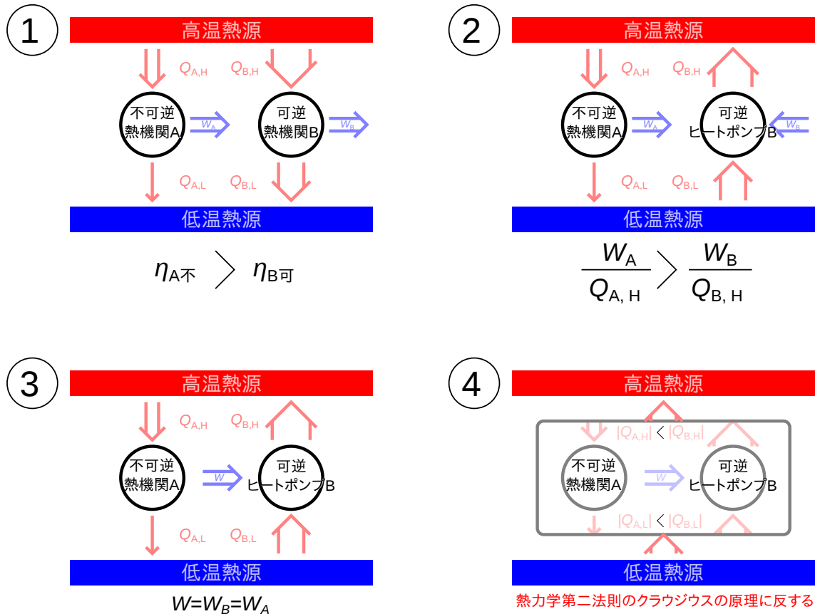
図 1.8 可逆熱機関と不可逆熱機関の比較
