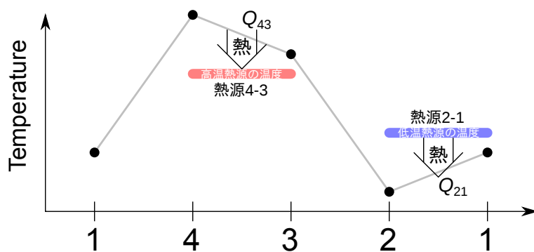
図 3.13 ピストンでのヒートポンプとして動作するサイクルの温度変化
