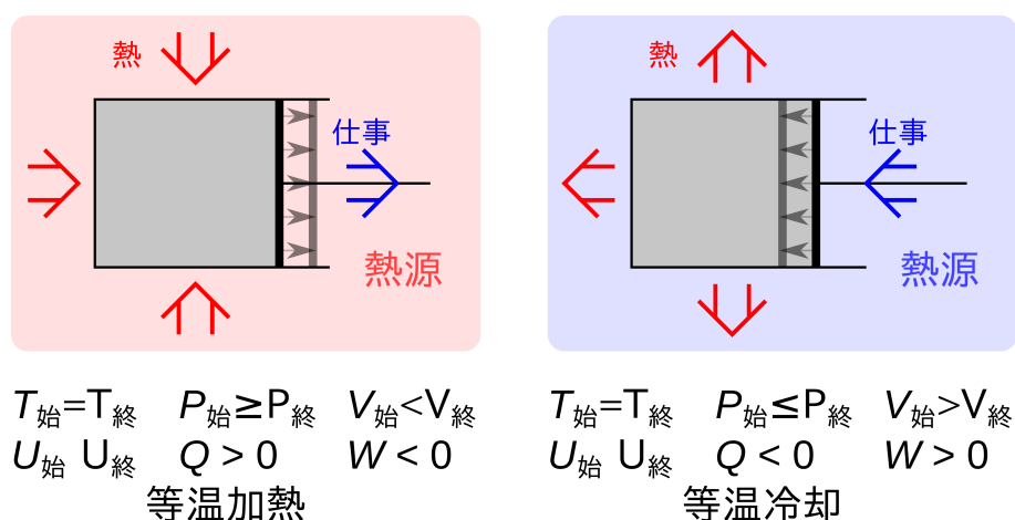
図 3.4 等温過程
