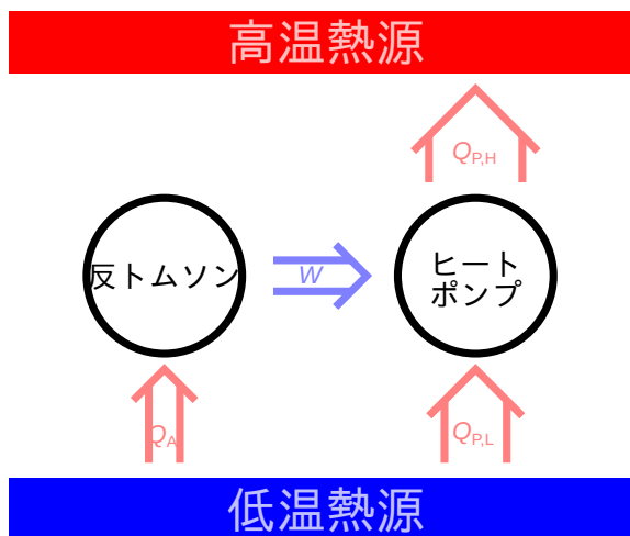
図 A.3 反トムソンの原理から反クラウジウスの原理
