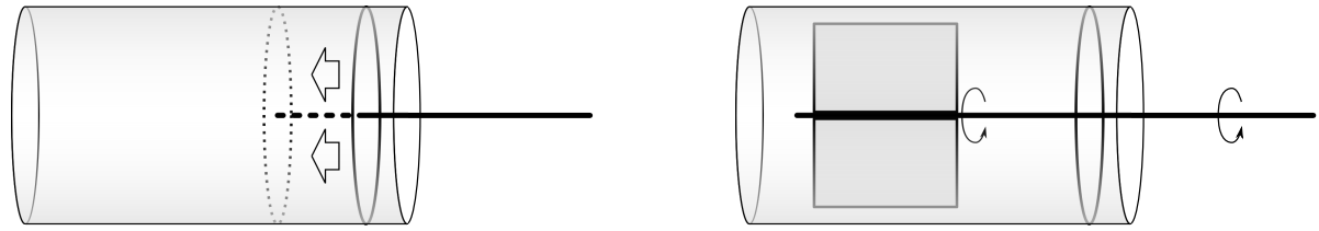
(a) 並進運動による仕事
