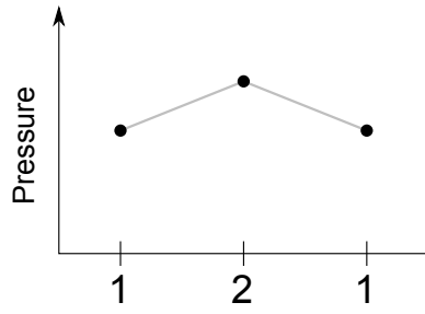
図 B.7 圧力変化
