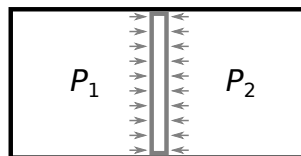
図 2.1 圧力と力学平衡
