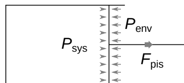
図 B.4 力の釣り合い（系の圧力が低い場合）
