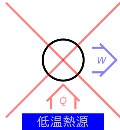
図 1.4 トムソンの原理
