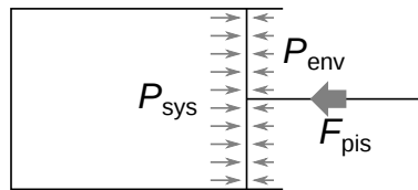
図 B.3 力の釣り合い（系の圧力が高い場合）
