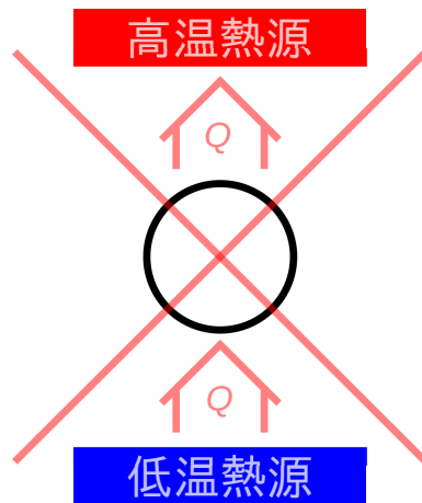
図 1.3 クラウジウスの原理
