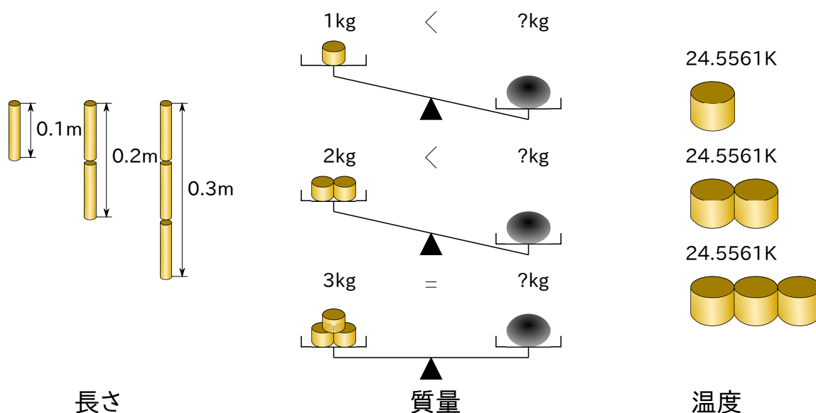
図 2.3 長さと質量と温度
