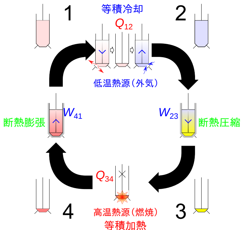
図 3.10 オットーサイクル
