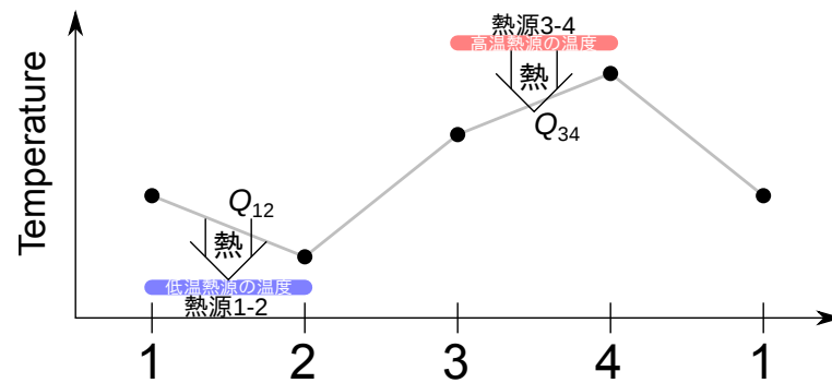
図 3.8 ピストンでの熱機関として動作するサイクルの温度変化
