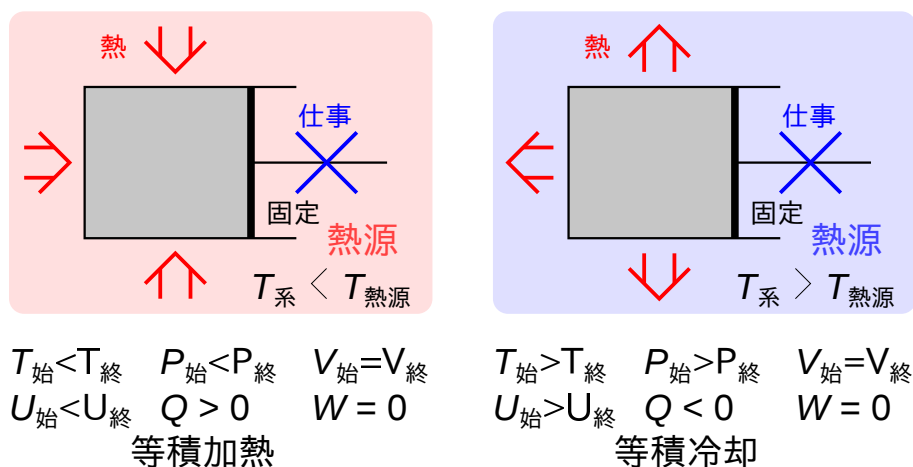
図 3.3 等積過程
