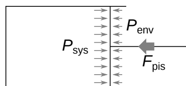
図 B.3 力の釣り合い（系の圧力が高い場合）
