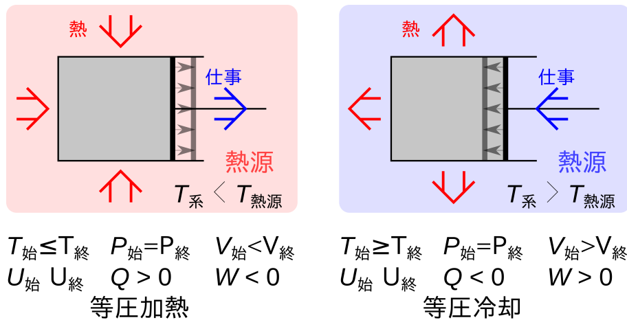
図 3.5 等圧過程
