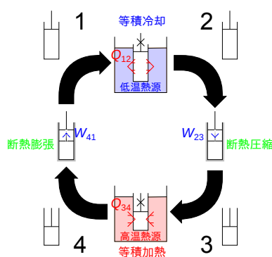
図 3.6 ピストンでの熱機関として動作するサイクル
