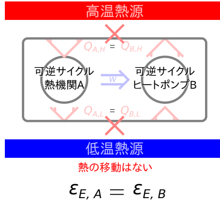
図 1.17 効率の等しい可逆サイクル
