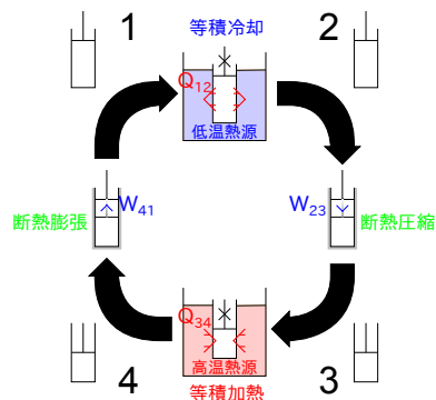
図 1.7 ピストンでの熱機関として動作するサイクル
