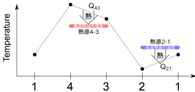
図 1.13 ピストンでのヒートポンプとして動作するサイクルの温度変化
