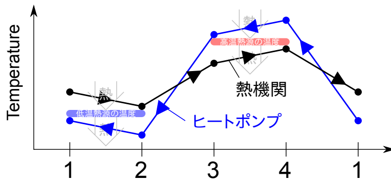
図 1.21 熱機関とヒートポンプにおける温度変化
