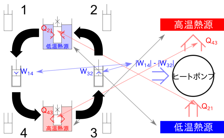
図 1.14 ヒートポンプの表示
