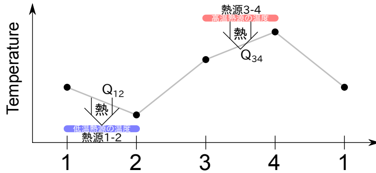
図 1.9 ピストンでの熱機関として動作するサイクルの温度変化
