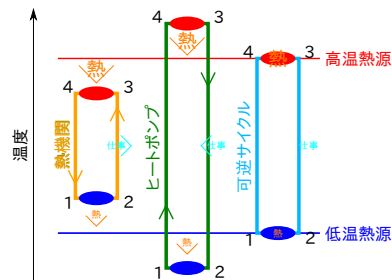
図 1.22 熱機関とヒートポンプにおける熱源との関係
