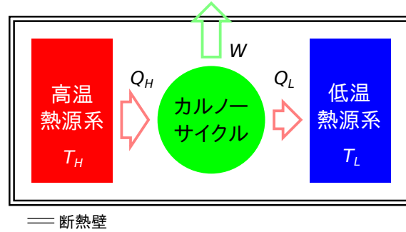
図 2.4 熱源とカルノーサイクル
