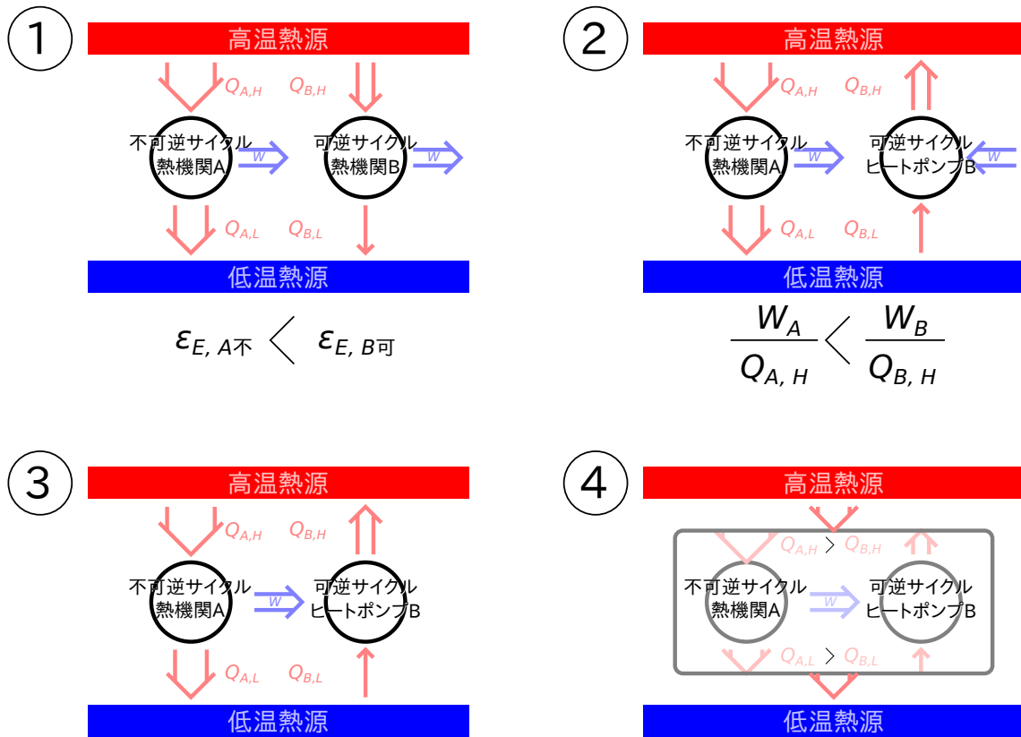
図 B.7 可逆サイクルと不可逆サイクルの比較
