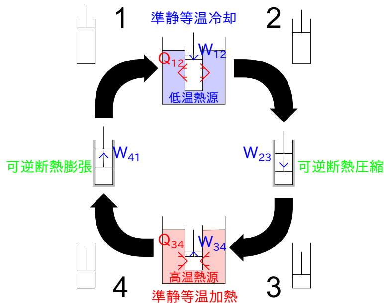
図 1.24 カルノーサイクル
