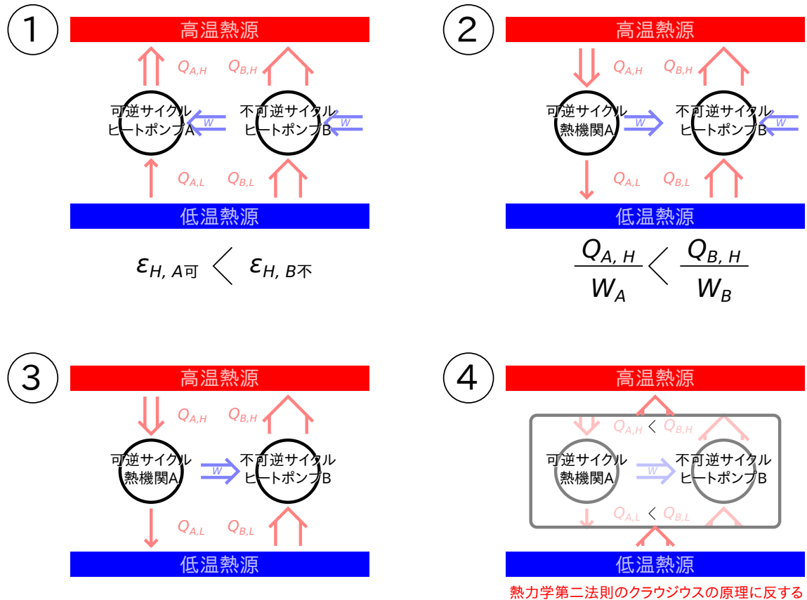
図 1.19 可逆サイクルのヒートポンプと不可逆サイクルのヒートポンプの比較
