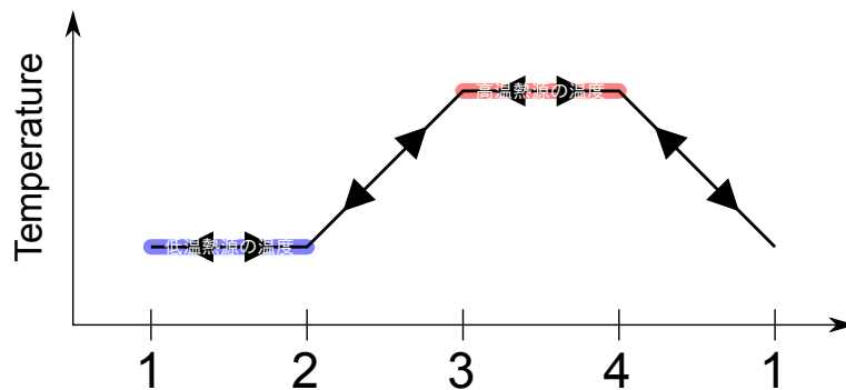
図 1.23 可逆サイクルにおける温度変化
