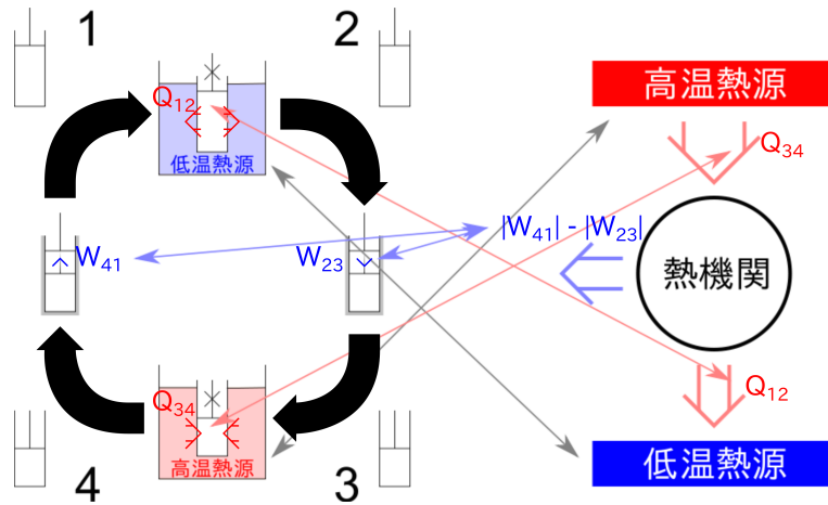
図 1.10 熱機関の表示
