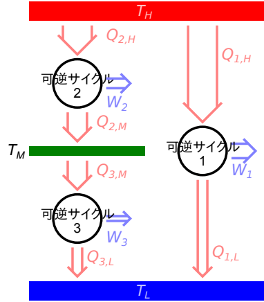
図 1.20 可逆サイクルの効率
