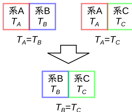
図 2.2 第零法則
