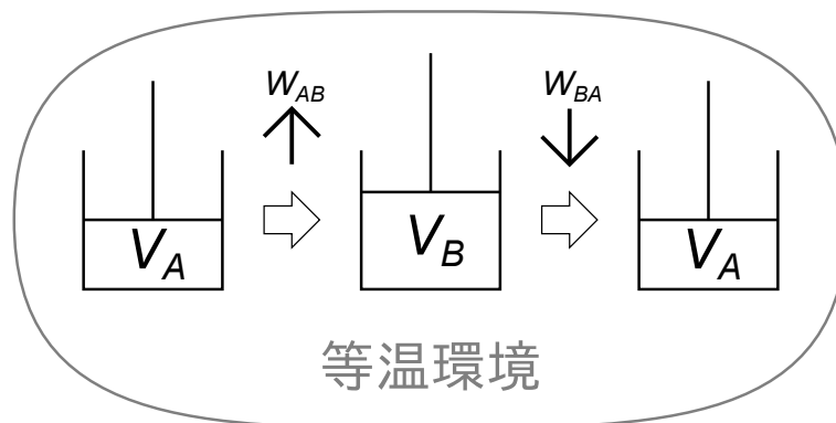
図 1.25 等温過程
