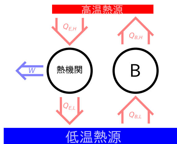
図 A.4 クラウジウスの原理
