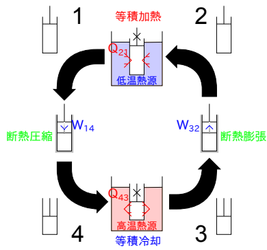
図 1.11 ピストンでのヒートポンプとして動作するサイクル
