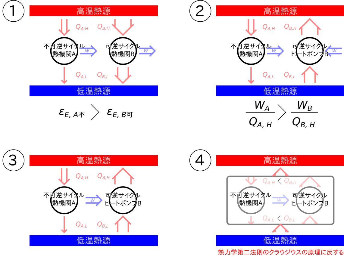
図 1.18 可逆サイクルと不可逆サイクルの比較
