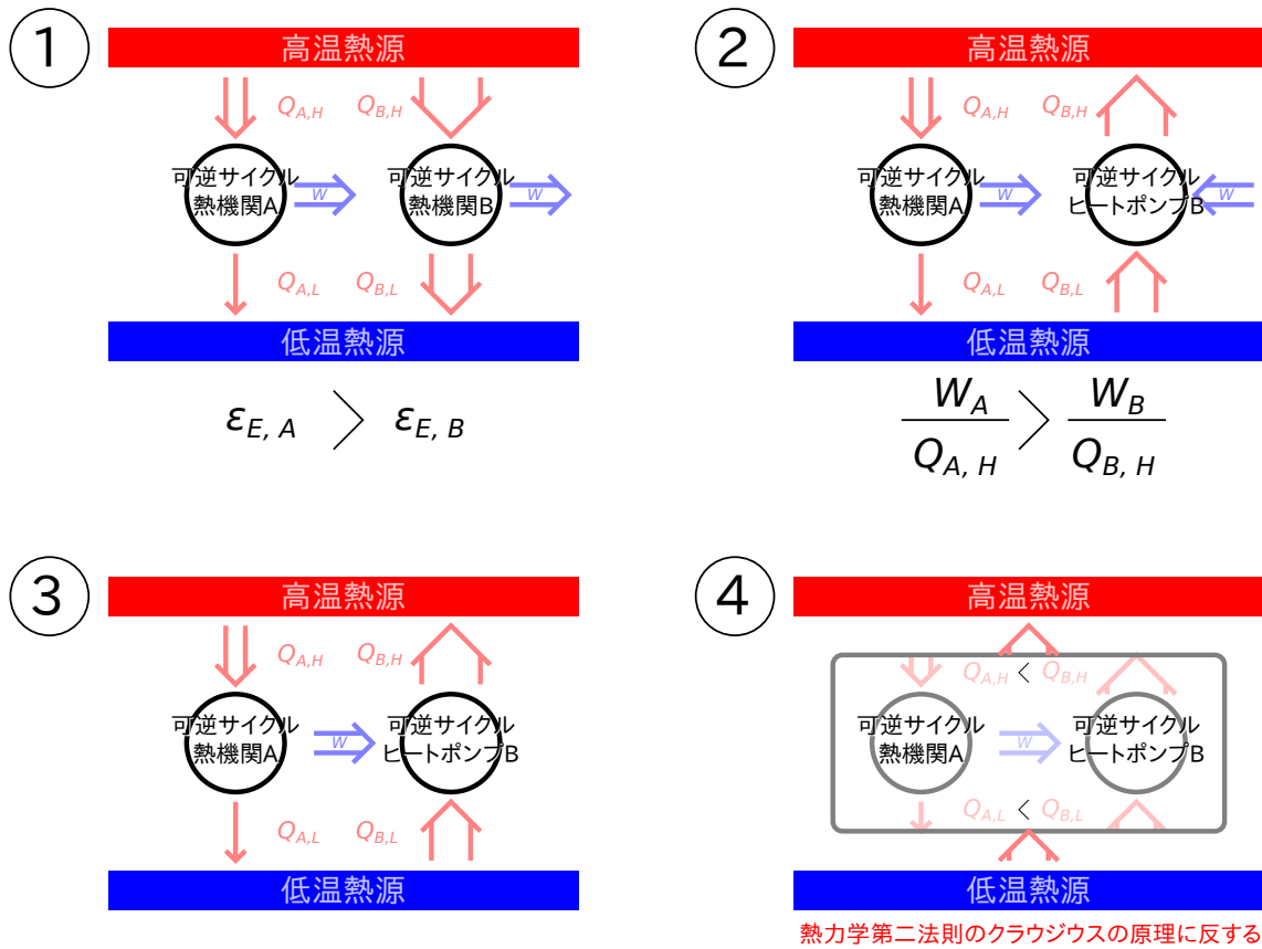
図 1.16 可逆サイクルの比較
