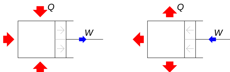
図 2.5 体積の変化する系
