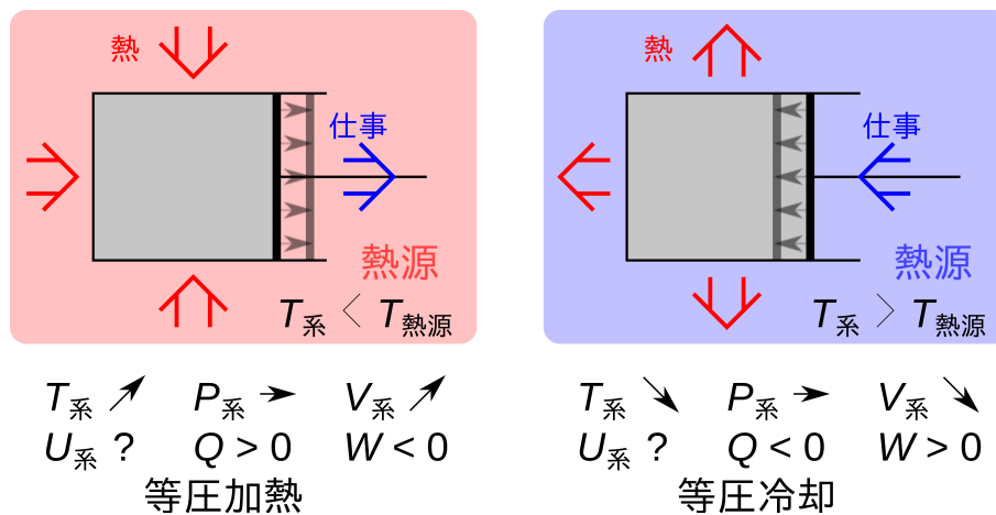
図 1.6 等圧過程
