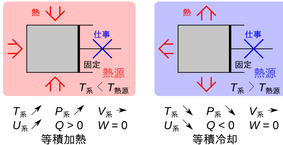
図 1.4 等積過程
