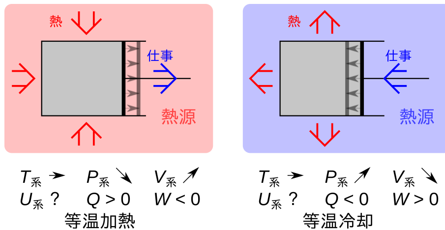
図 1.5 等温過程
